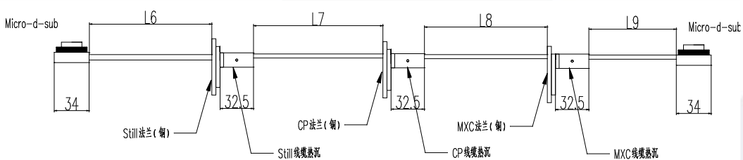
4K到MXC直流线尺寸图
