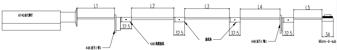
室温到4K直流线尺寸图
