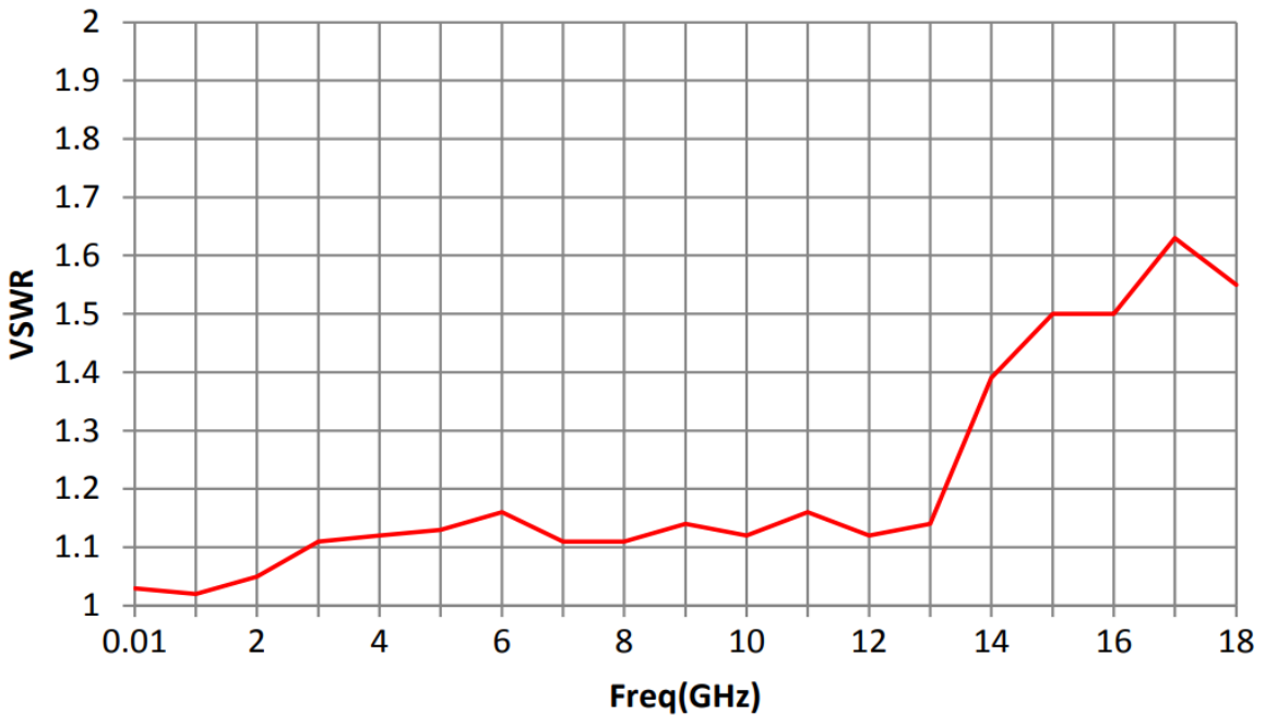
驻波比 VS 频率
