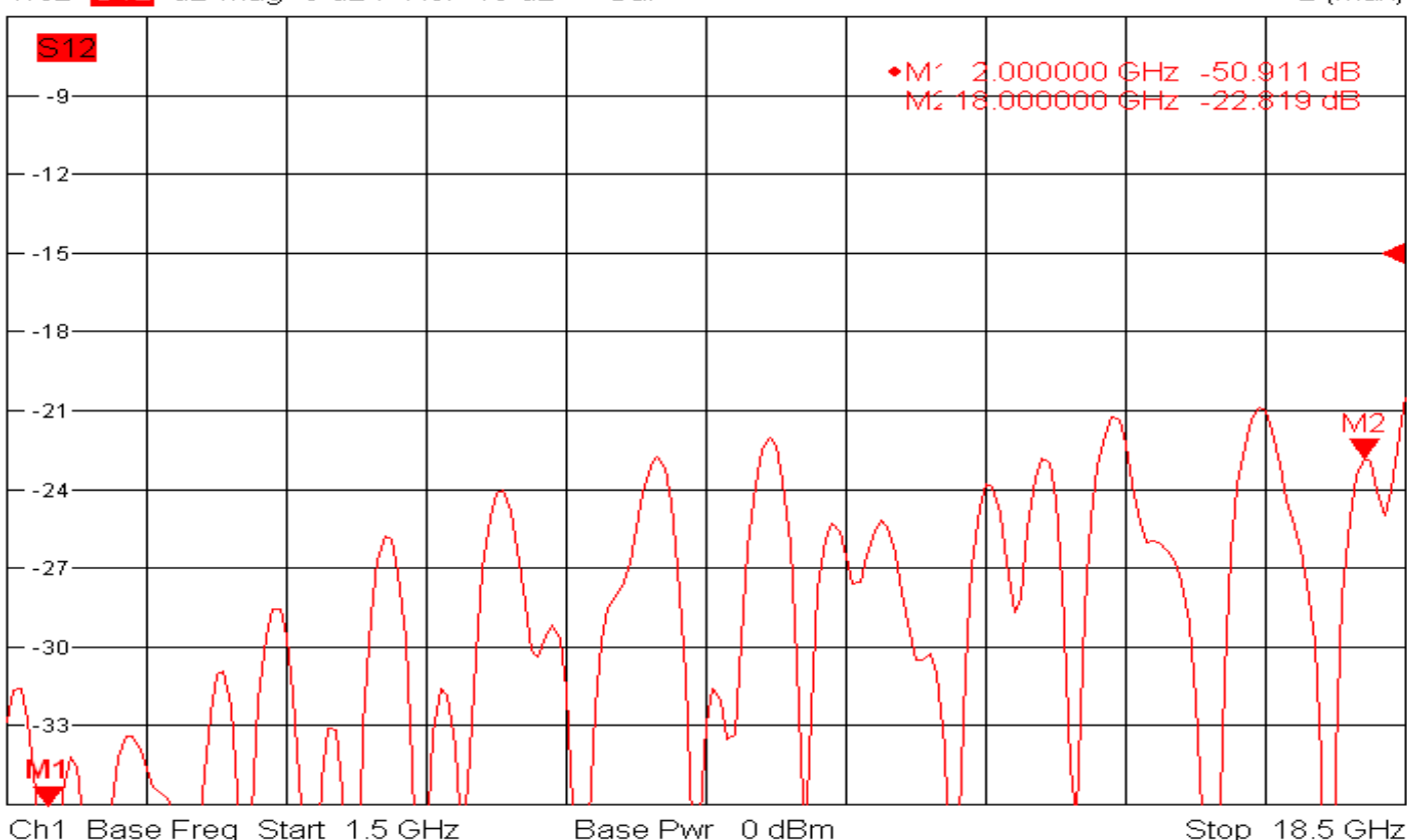
Trc2 S12 dB Mag 3 dB / Ref-15 dB Cal
