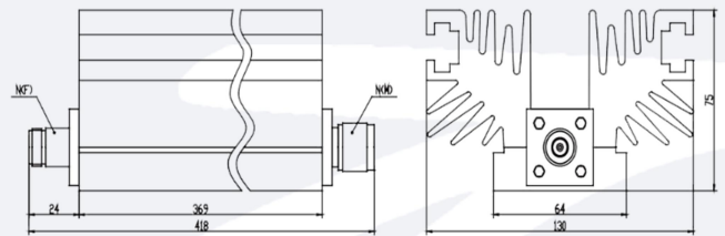
Unit:mm
